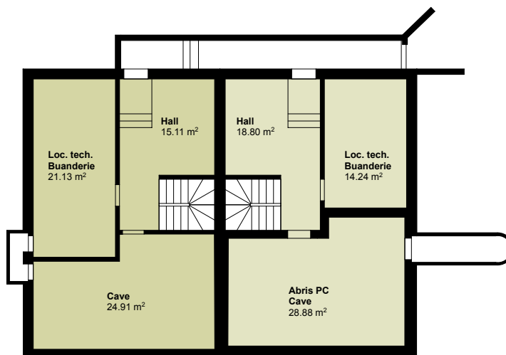
SOUS-SOL
